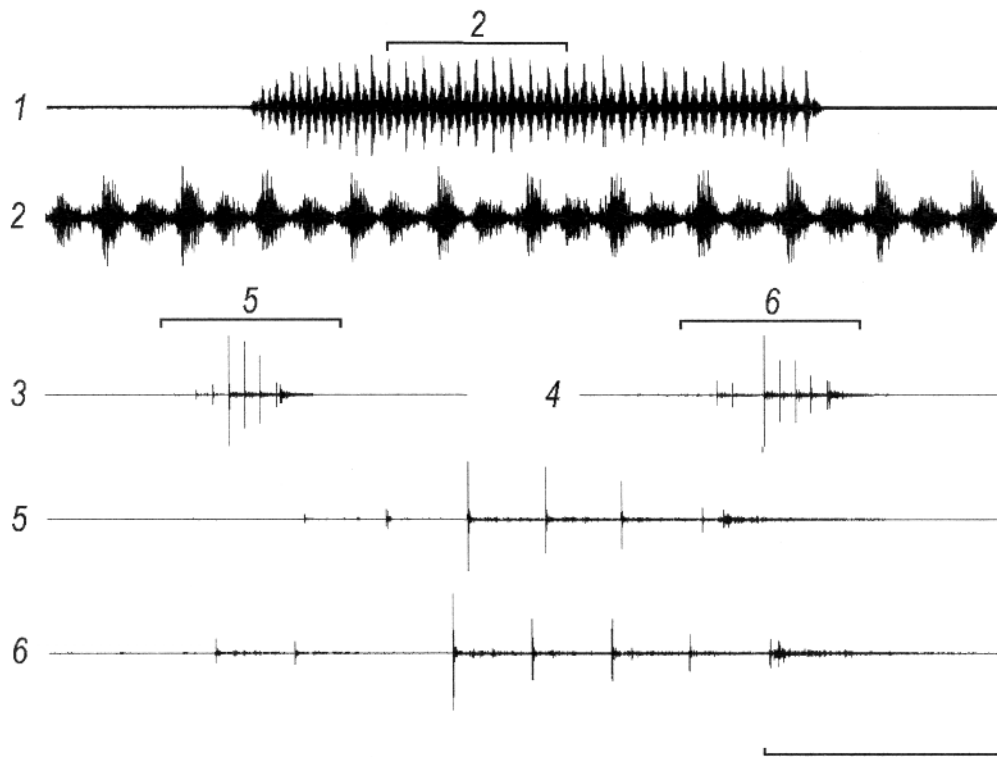
Рис. 2. Осциллограммы звуковых сигналов самцов Acrida bicolor (Thnb.), издаваемых тегмино-феморальным акустическим аппаратом (1-2) и в полете (3-6) при разной временной развертке. 1-2 — одиночный самец с одной правой задней ногой; 3-6 — в полете после вспугивания. Отметка времени внизу для осциллограмм 1, 3, 4 — 500 мс; 2, 5, 6 — 100 мс
